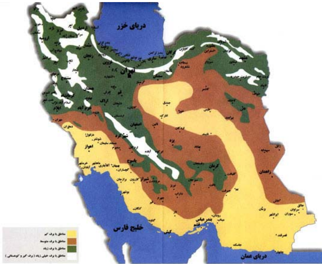
شکل ۶-۴- تقسیم بندی مناطق کشور برای بار برف
