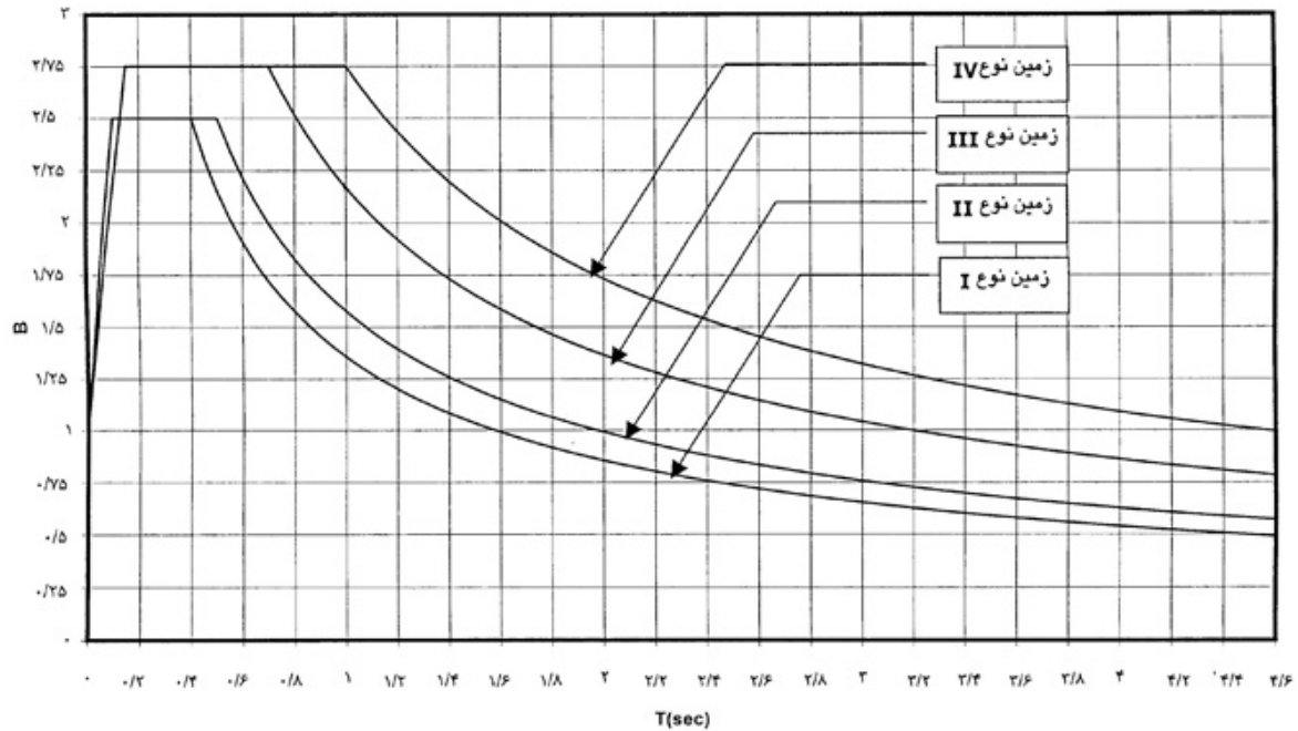
شکل ۶-۷-۱-ب - ضریب بازتاب ساختمان برای مناطق با خطر نسبی زیاد و خیلی زیاد
