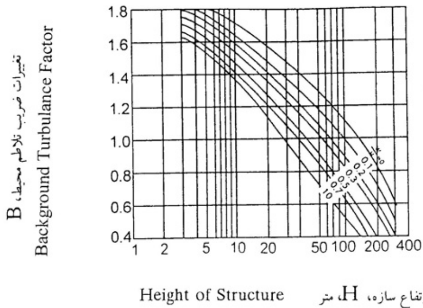
شکل پ - ۱ - ۳ - ۶ تغییرات ضریب تلاطم محیط با ابعاد سازه
