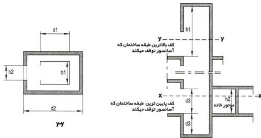
مقطع عمودی چاه و موتور خانه
