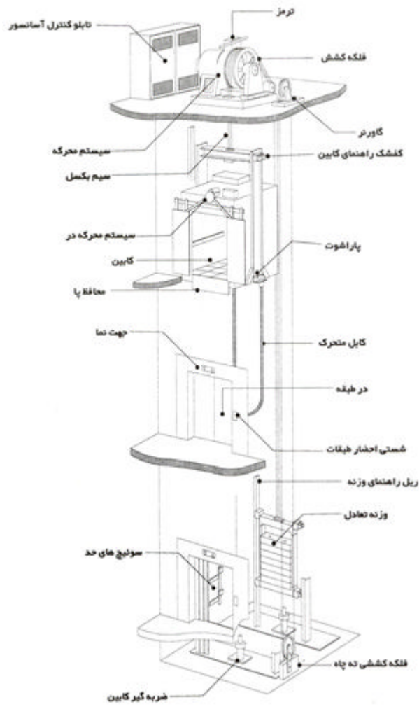
شکل ۱۵-۲-۱ اجزای آسانسور کششی
