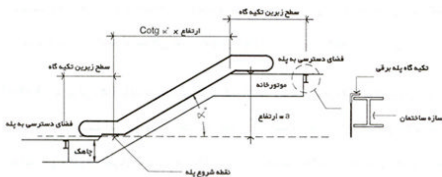
شکل ۱-۳-۱۵ طرح کلی پله برقی
