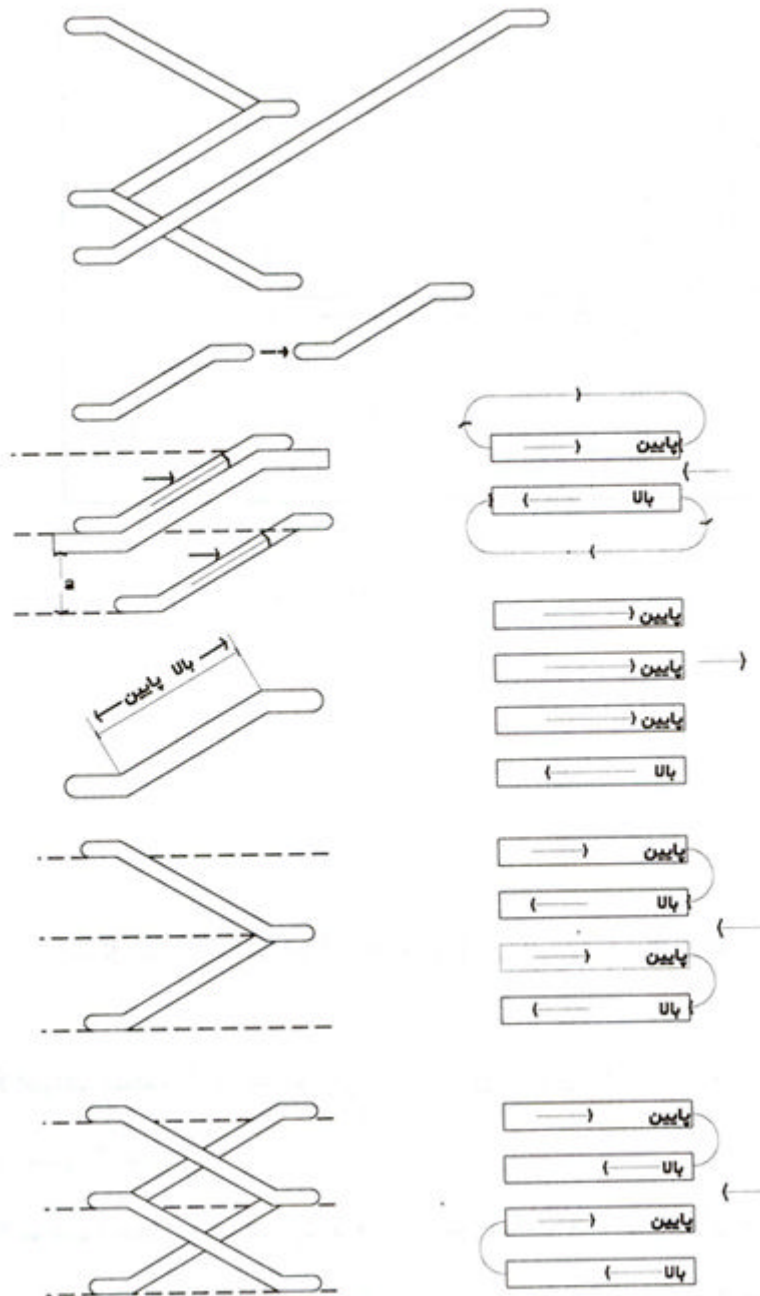
شکل ۳-۴-۱۵ آرایشهای مختلف پله برقی
