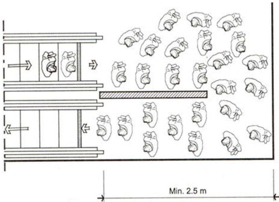
شکل ۱۵-۲-۴-۲ فضای باز در ورودی یا خروجی پله برقی
