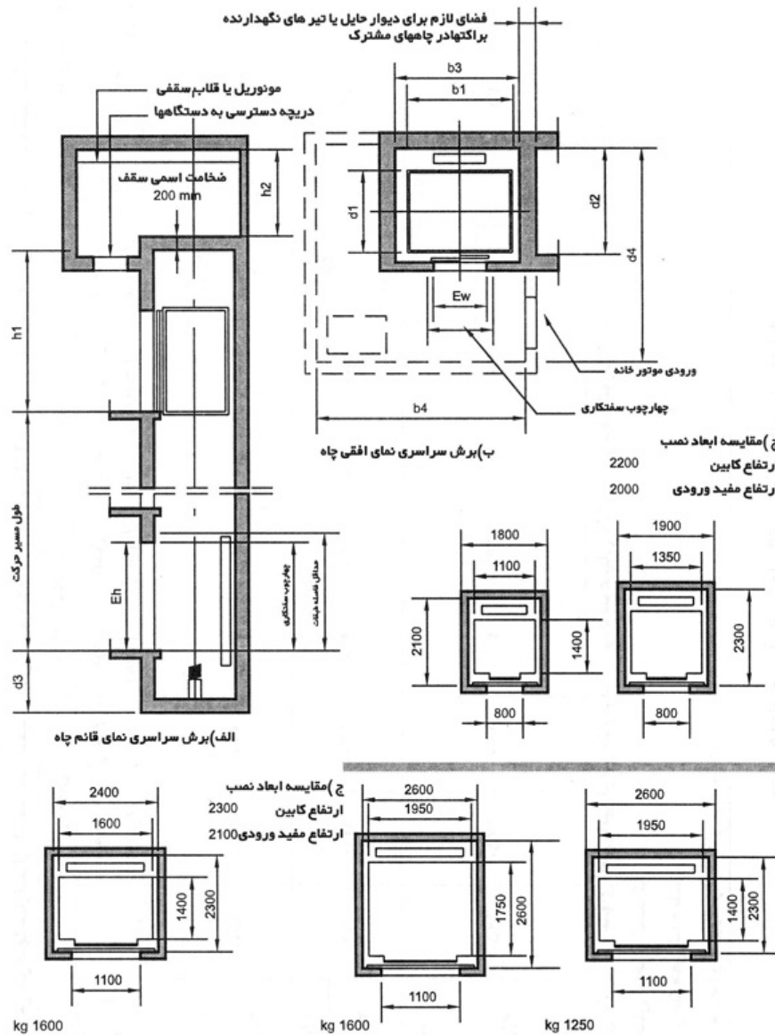
شکل ۲- طرح اولیه معماری آسانسورهای الکتریکی مسافری با کاربرد عمومی
