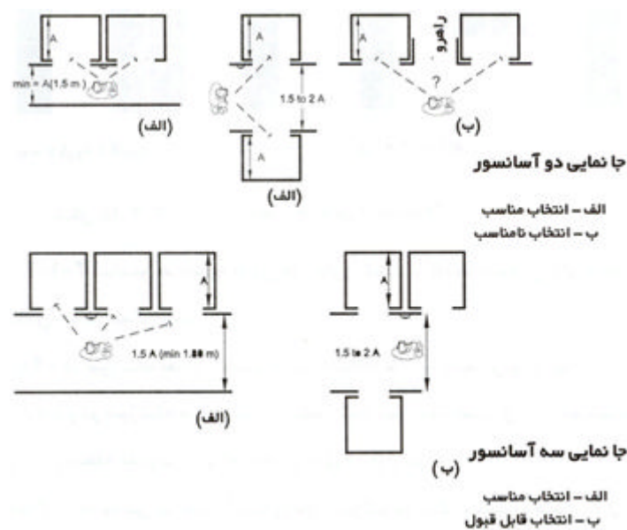
شکل ۴-۱-۲-۲-۱۵(الف) فضاهای انتظار راهروهای مقابل آسانسورها
