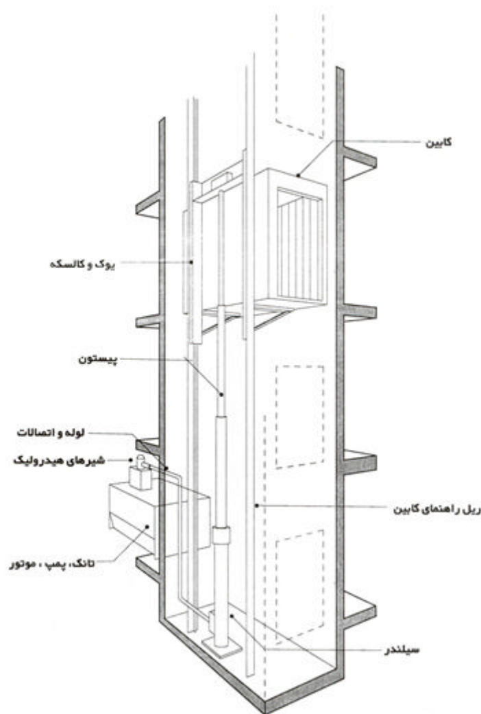
شکل ۱۵-۲-۱ اجزاء آسانسور هیدرولیک، سیستم مستقیم - کنار
