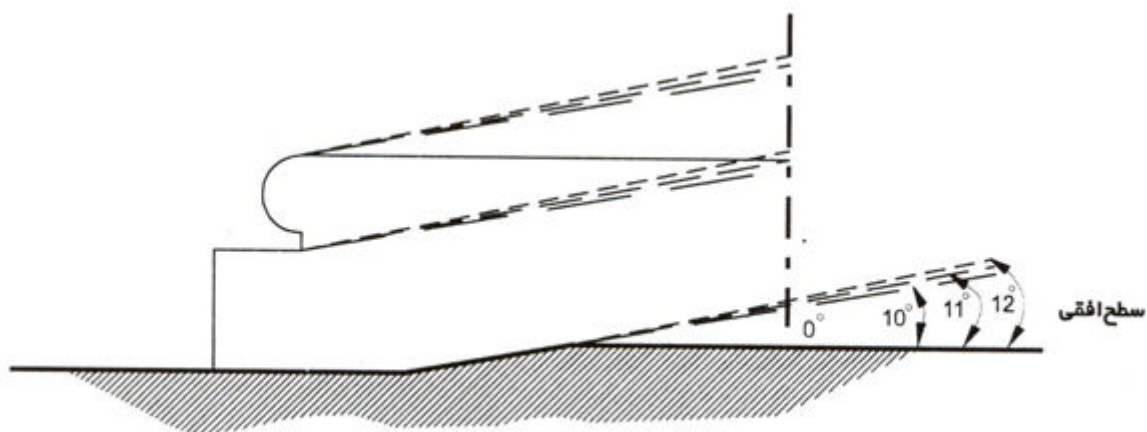
شکل ۱۵-۴-۲ زوایای شیب پیاده روهای متحرک
