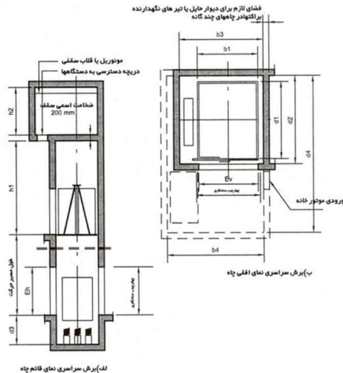
شکل ۷- طرح اولیه معماری آسانسورهای الکتریکی باری با کاربرد عمومی
