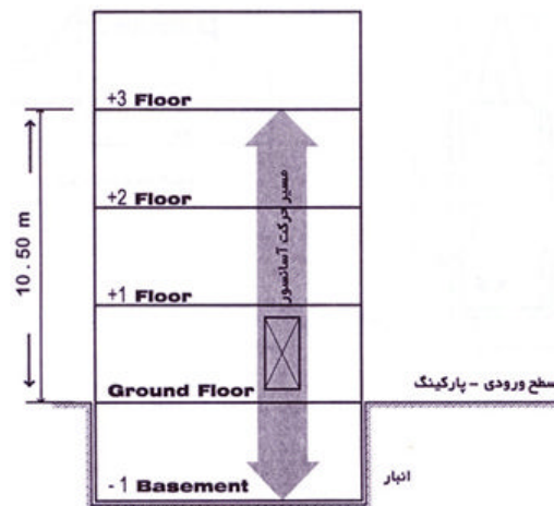
شکل ۹- تعیین حداکثر ارتفاع
