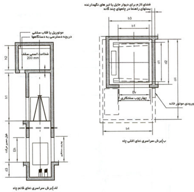
شکل ۸- طرح اولیه معماری آسانسورهای الکتریکی باری سنگین
