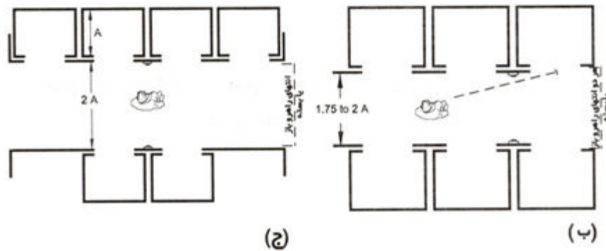
شکل ۱۵-۲-۲-۱-۴ (ب) فضاهای انتظار در راهروهای مقابل آسانسورها
