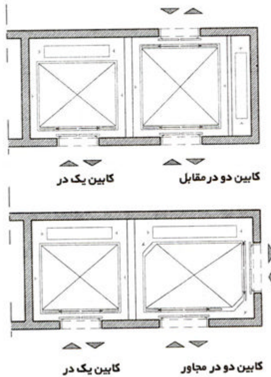
شکل ۴-۱-۲-۱۵ کابین دو در مقابل - دو در مجاور
