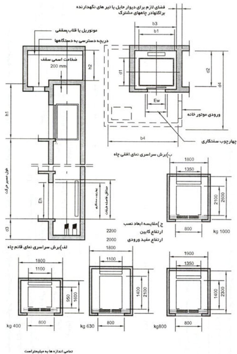
شکل ۱-۲ طرح اولیه معماری آسانسورهای الکتریکی ساختمانهای مسکونی
