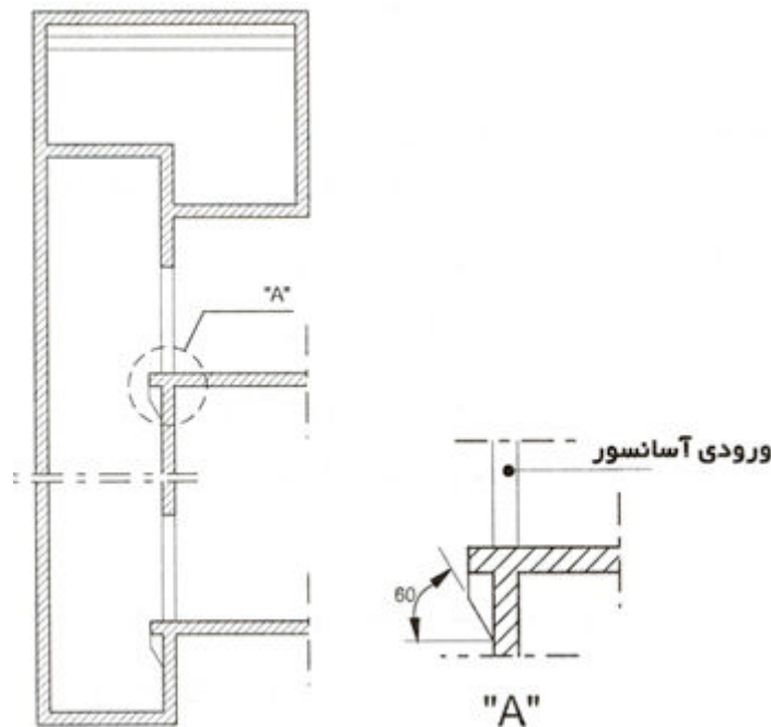
شکل ۴-۳-۲-۲-۱۵ سطح داخلی دیواره چاه در سمت ورودی طبقات
