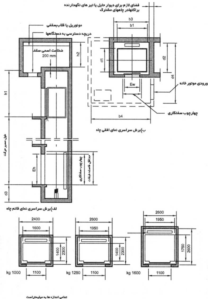
شکل ۵- طرح اولیه معماری آسانسور های الکتریکی مسافری بانرد زباده
