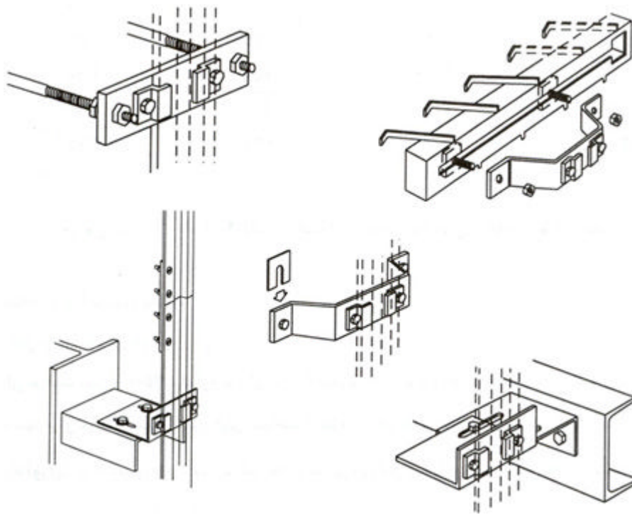
۱۵-۲-۲-۱ انواع براکت و نحوه اتصال به سازه های فلزی و بتنی
