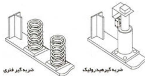
شکل ۱۵-۲-۳ دو نوع ضربه گیر کف چاهک
