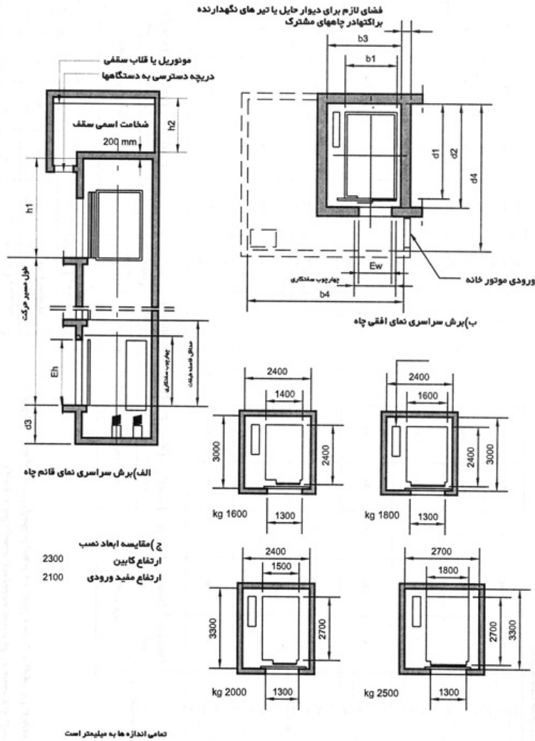
شکل ۶- طرح اولیه معماری آسانسورهای الکتریکی حمل تخت بیمار و مسافر
