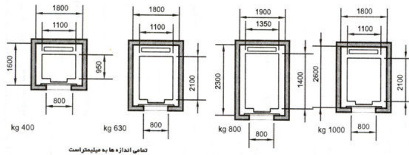
شکل ۱-۲ طرح اولیه معماری آسانسورهای الکتریکی با تردد کم
