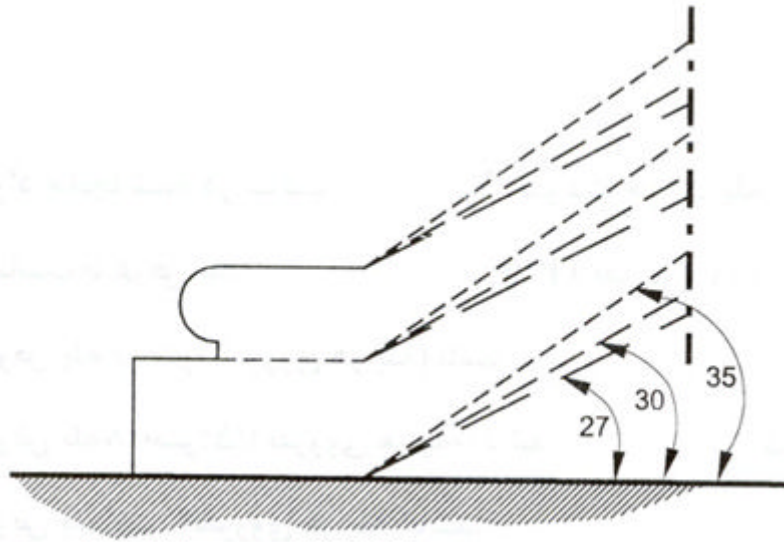
شکل ۱۵-۲-۹-۴ زوایای شیب پله برقی
