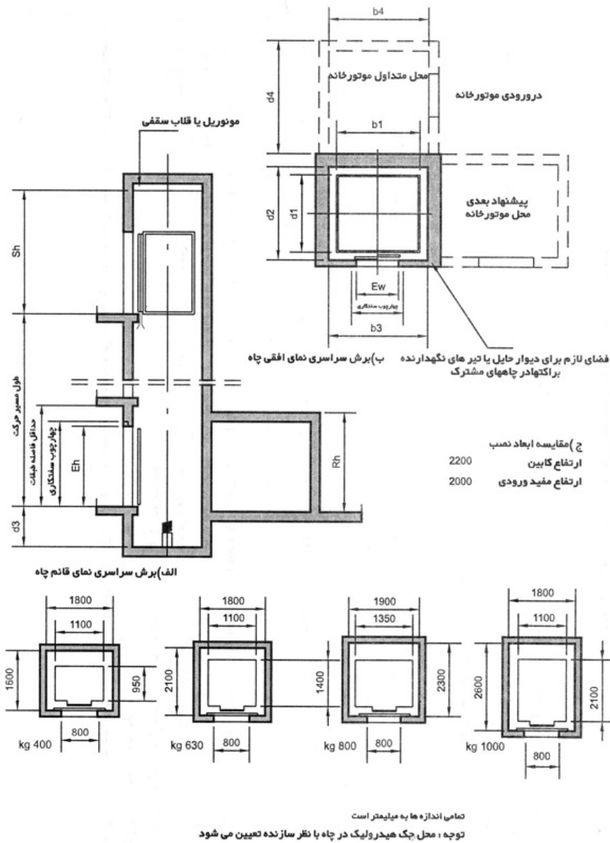
شکل ۲-۲ طرح اولیه معماری آسانسورهای هیدرولیکی مسافری با تردد کم
