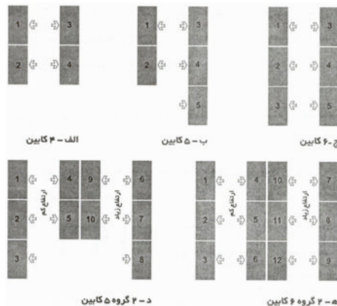
شکل ۱-۱-۲-۲-۱۵ نمونه های جانمایی آسانسورها
