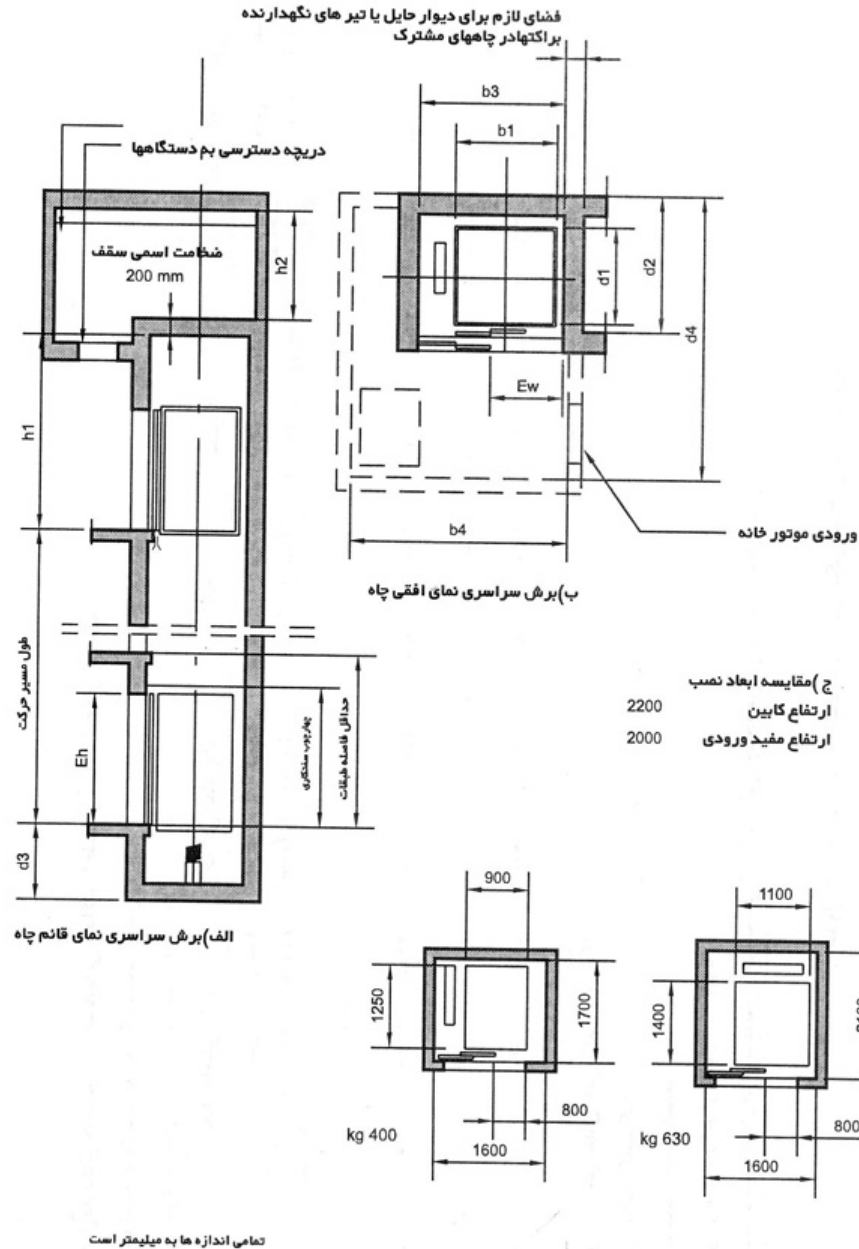
شکل ۳-۲- طرح اولیه معماری آسانسورهای الکتریکی مسافری با تردد موردی
