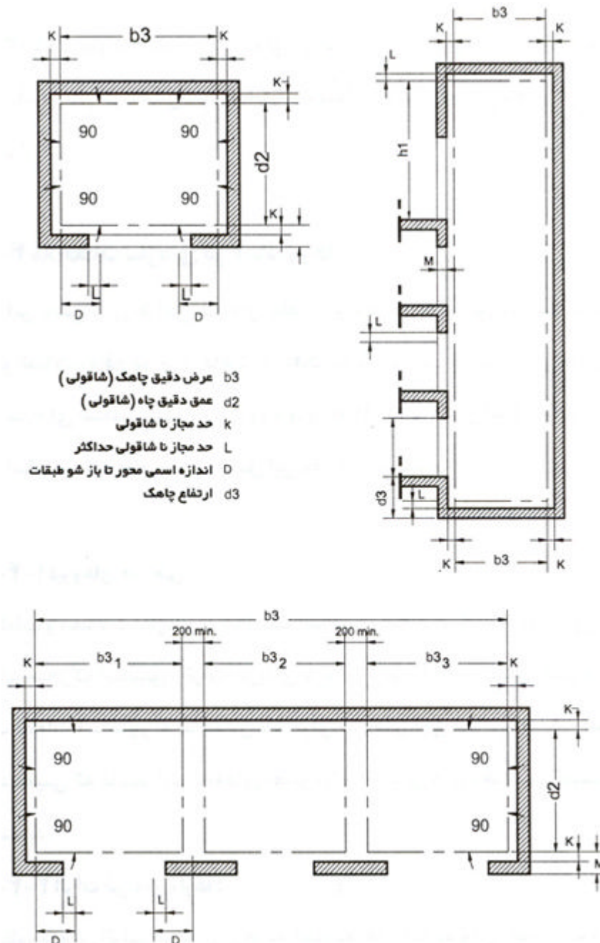
شکل ۲-۹-۲-۲-۱۵ خطوط شاقولی و دیواره‌های جداساز چاه‌های آسانسور
